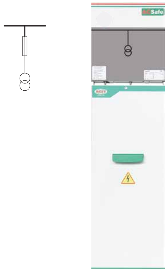
Chiều rộng / width: 800mm Chiều sâu / depth: 1000mm Chiều cao / height: 1375mm
