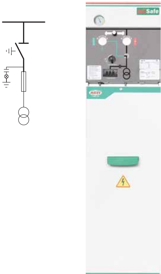
Chiều rộng / width: 600mm Chiều sâu / depth: 800mm Chiều cao / height: 1375mm
