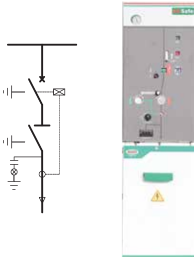
Chiều rộng / width: 375mm Chiều sâu / depth: 800mm Chiều cao / height: 1375mm
